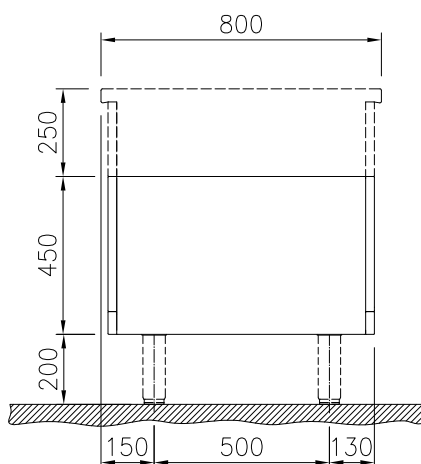
Boven aanzicht
